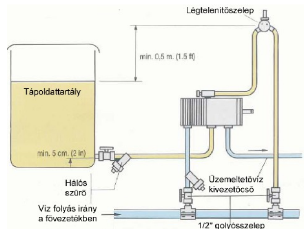
Ecofertic csatlakozási vázlat.
