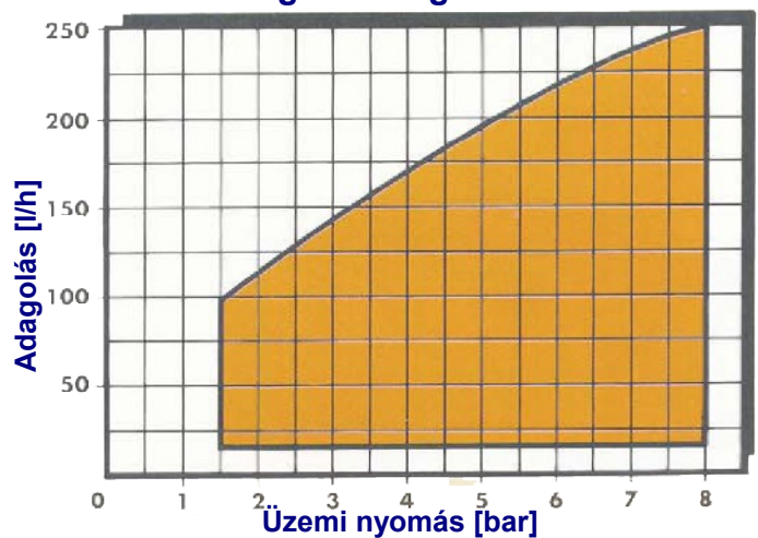
Ecofertic adagolás diagrama.
