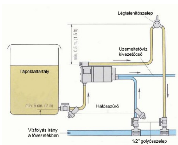
Fertic csatlakozási vázlatja.
